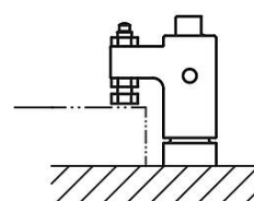
3. Fixieren der Spannschraube mittels Sechskantmutter.
