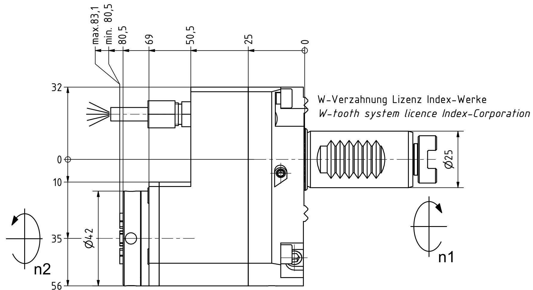
Spannzange / Collet ER16 DIN6499 Spannbereich / Clamping range: 1,0 - 10,0
