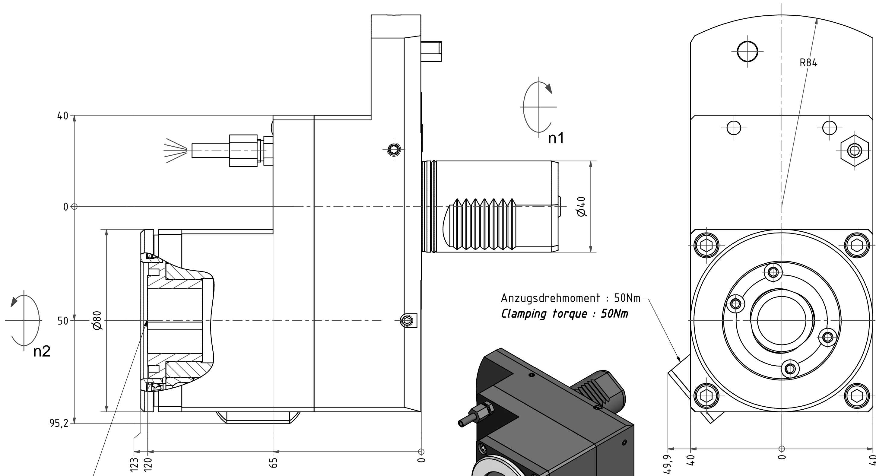
Capto C4-Aufnahme Capto C4-Adaptor
